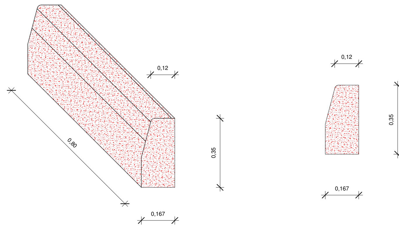
14 DETALHE MEIO FIO 1 : 10
