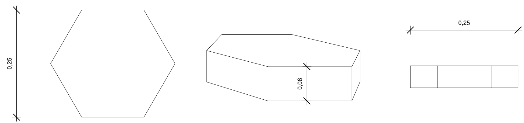
17 Detalhe 01 Bloco Sextavado 1 : 5
