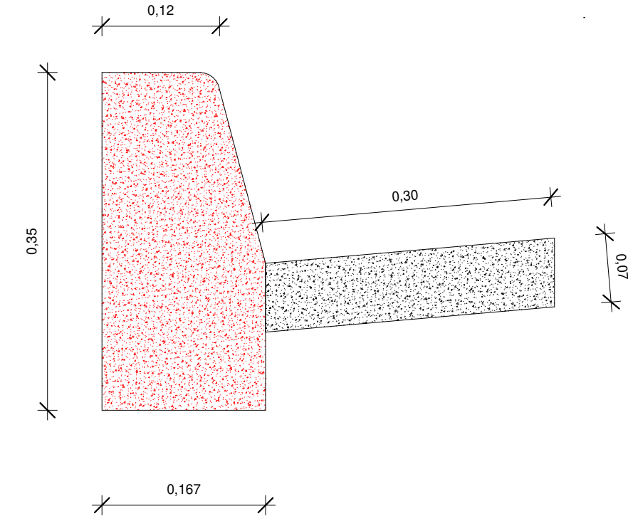
19 Guia Mei-Fio e Sarjeta 1 : 5
