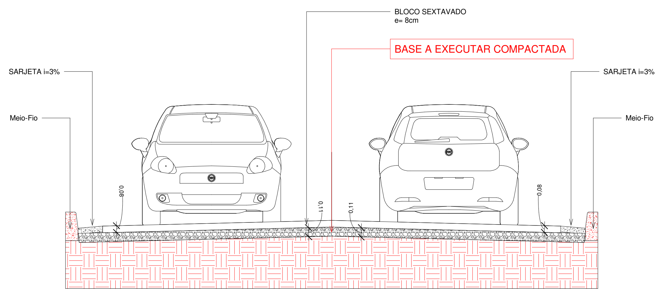
15 Pista de Rolamento 1 : 25
