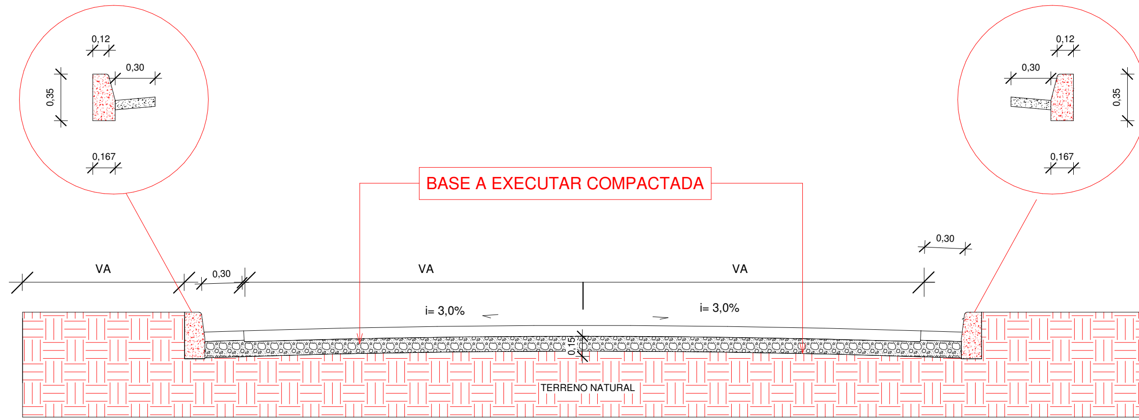
20 CORTE TRANSVERSAL 1 : 25
